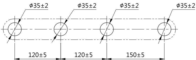
龍頭挖孔尺寸
