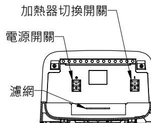
A-A 斷面圖 (由下往上看)
