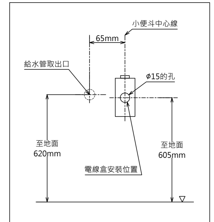
電源盒安裝位置(示意圖)
