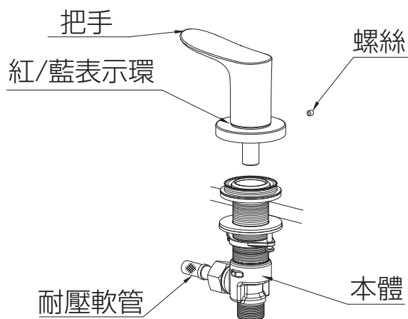
圖4(把手的安裝)
