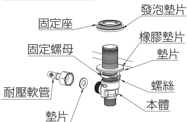
圖2(本體的安裝)
