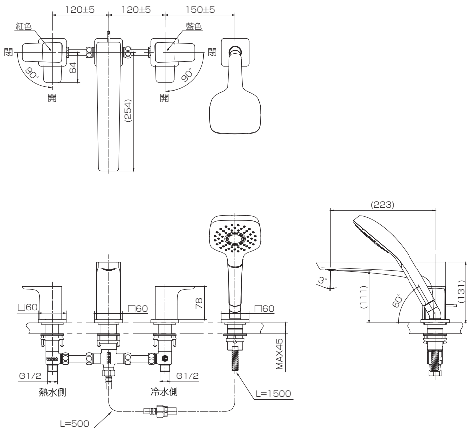
浴缸用四孔混合龍頭 (附一段式蓮蓬頭) 例：TBG07202P
