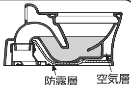
<參考>防露馬桶·水箱的構造
